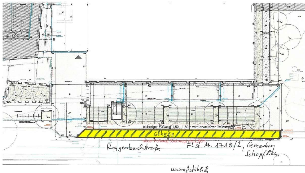
Planung Schulcampus Schopfheim – Stand März 2022 Freianlagen vor der neuen Sporthalle mit neuen Parkflächen und Fußweg
